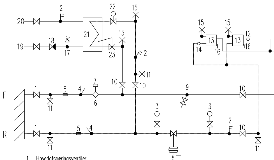
PRINCIPDIAGRAM
